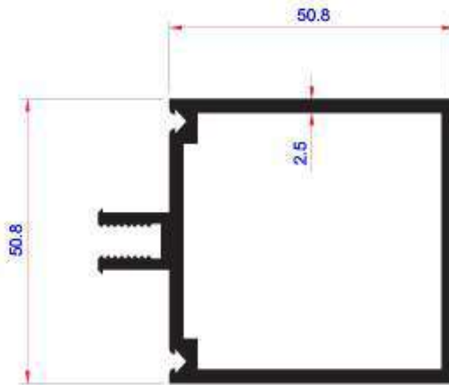
12395 1.499 kg/m
