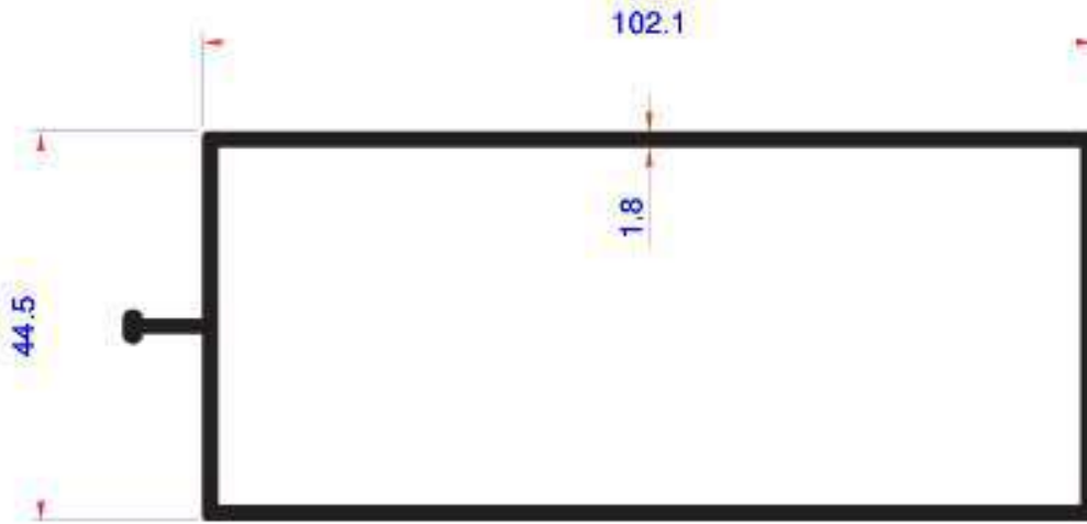
12406 1.450 kg/m
