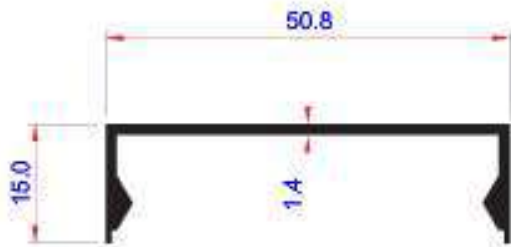
12908 0.327 kg/m
