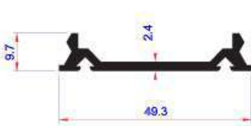
12907 0.435 kg/m
